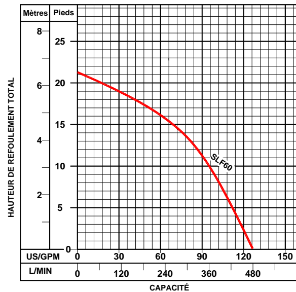
COURBE POMPAGE SÉRIE SLF
