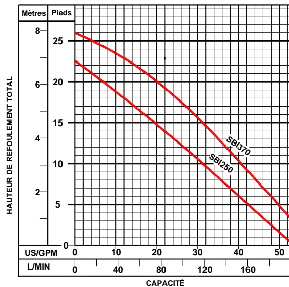
COURBE POMPAGE SÉRIE SBI
