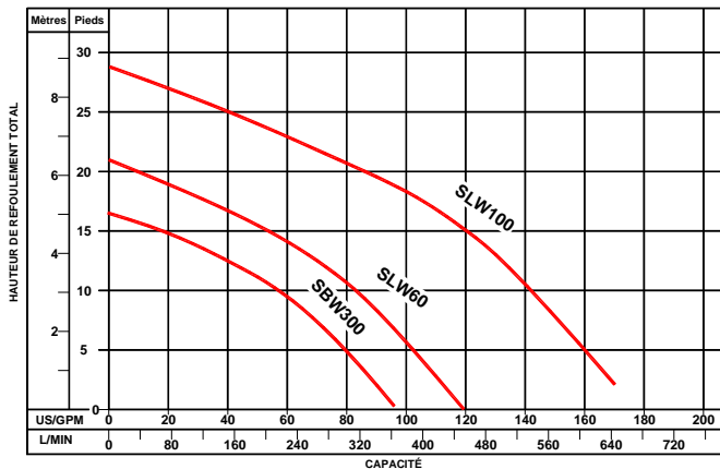
COURBE POMPAGE SÉRIE SBW / SLW
